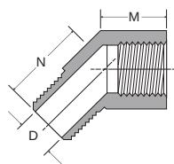
2214P - Cotovelo 45° macho-fêmea NPTF
