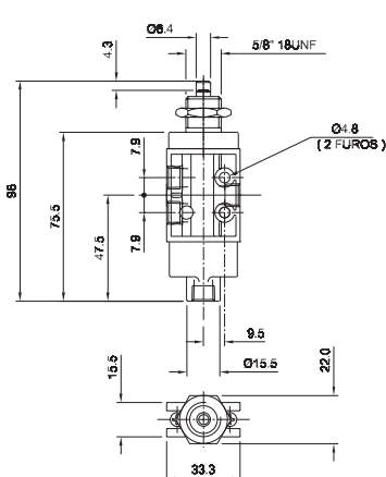
Válvula pino/piloto - 3/2 vias
