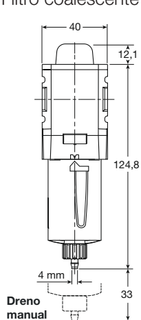
Filtro coalescente
