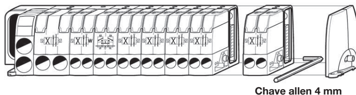
Série V montagem da ilha básica (sem conexões)
