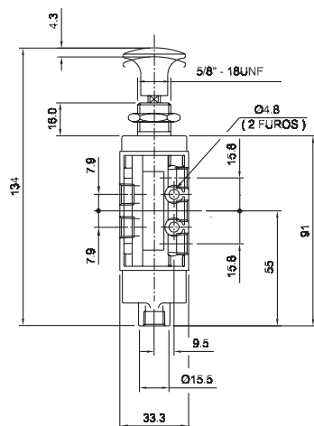
Válvula botão/piloto - 5/2 vias
