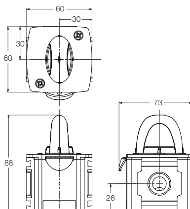
P32VB - G 1/2"
