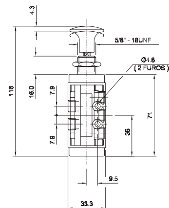
Válvula botão/piloto - 3/2 vias
