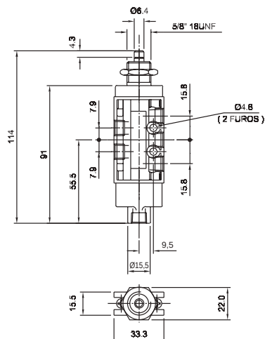
Válvula botão/trava - 3/2 vias
