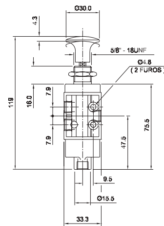
Válvula alavanca/trava - 5/2 vias
