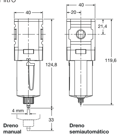
Filtro
