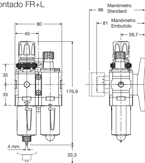
Conjunto montado FR+L
