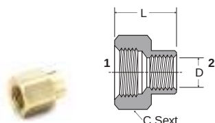
208P - Luva redução NPTF / SAE 130138
