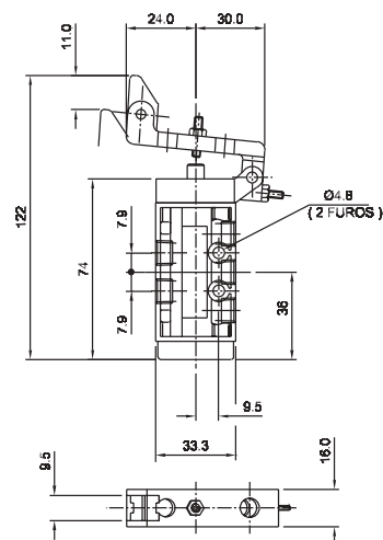
Válvula pino/piloto - 3/2 vias
