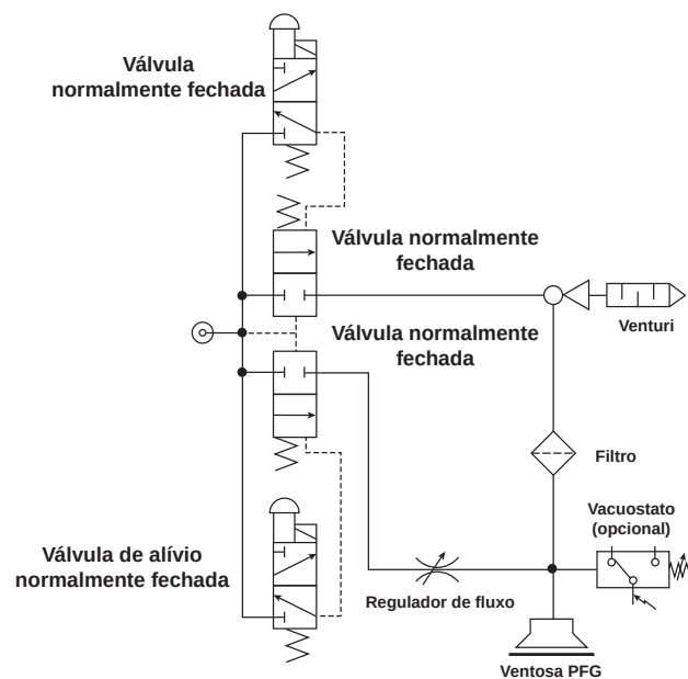
Normalmente fechado
