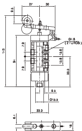
Válvula pino/mola - 3/2 vias
