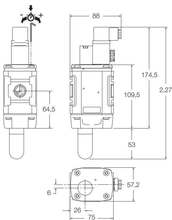
P32TA - 1/2"
