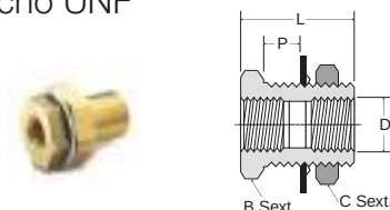
207ACBH - Junta de acoplamento Fêmea NPTF / macho UNF
