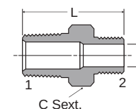
216P - Niple redução sextavado NPTF
