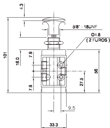
Válvula botão/piloto - 5/2 vias
