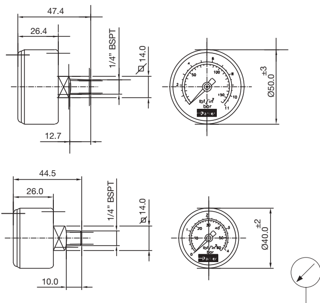
Manômetro versão normal
