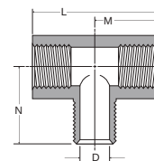
2224P - Tê macho-fêmea rosca central NPTF / SAE 130425
