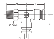
W171PLP - Tê macho lateral orientável Tubo / macho NPTF
