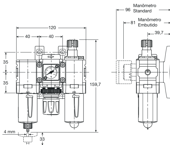
Conjunto montado F+R+L
