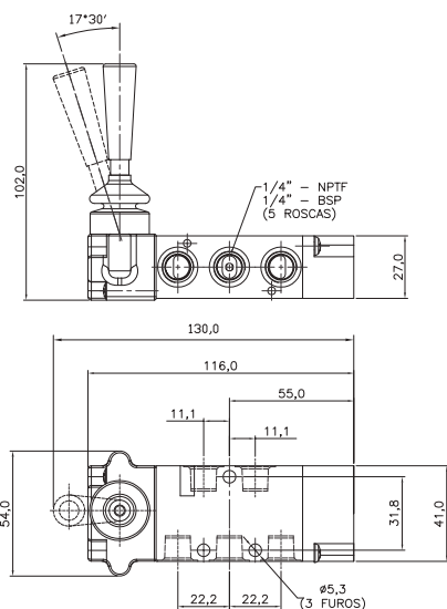
Válvula alavanca/mola
