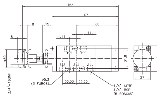
Válvula botão autocentrante para painel (3 posições)
