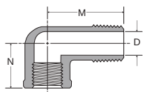
1202P - Cotovelo 90° macho-fêmea NPTF
