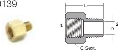
222P - Adaptador macho-fêmea NPTF / SAE 130139
