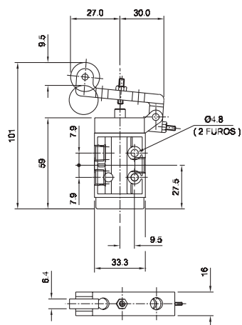
Válvula rolete/piloto - 5/2 vias
