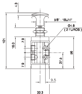
Válvula botão/trava - 5/2 vias
