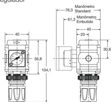
Regulador
