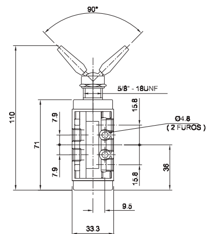
Válvula alavanca/trava - 5/2 vias
