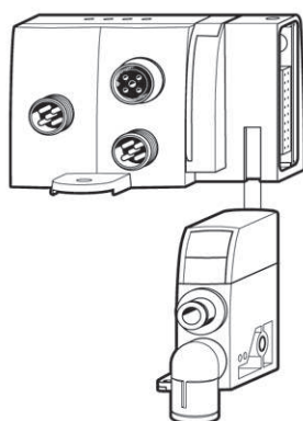
① Montagem do módulo de comunicação e alimentação pneumática
