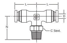
W172PLP - Tê macho central orientável Tubo / macho NPTF
